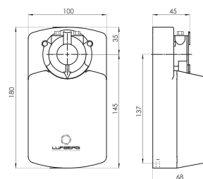
РАЗМЕРЫ (мм)
